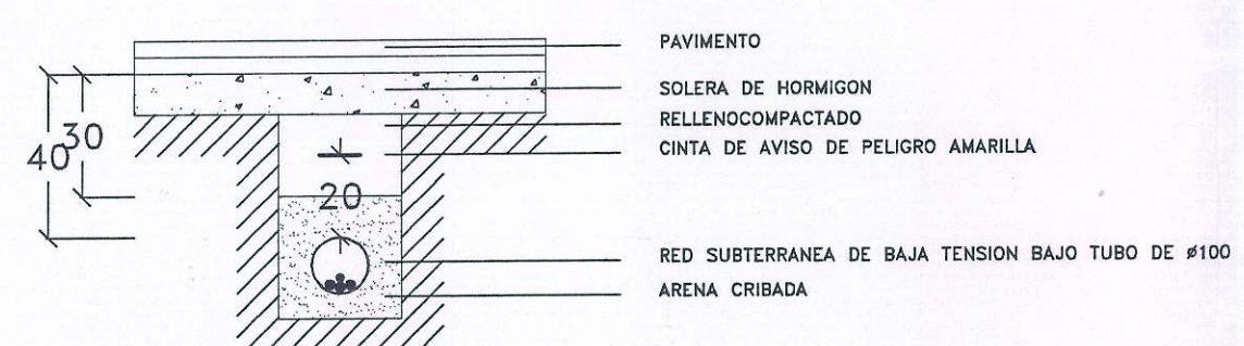
ALUMBRADO CANALIZACION BAJO ACERA. 1:20. COTAS EN CM.
