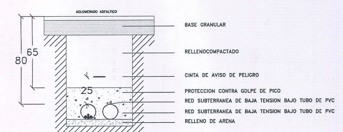
ALUMBRADO. CANALIZACION BAJO CALZADA. 1:20. COTAS EN CM.
