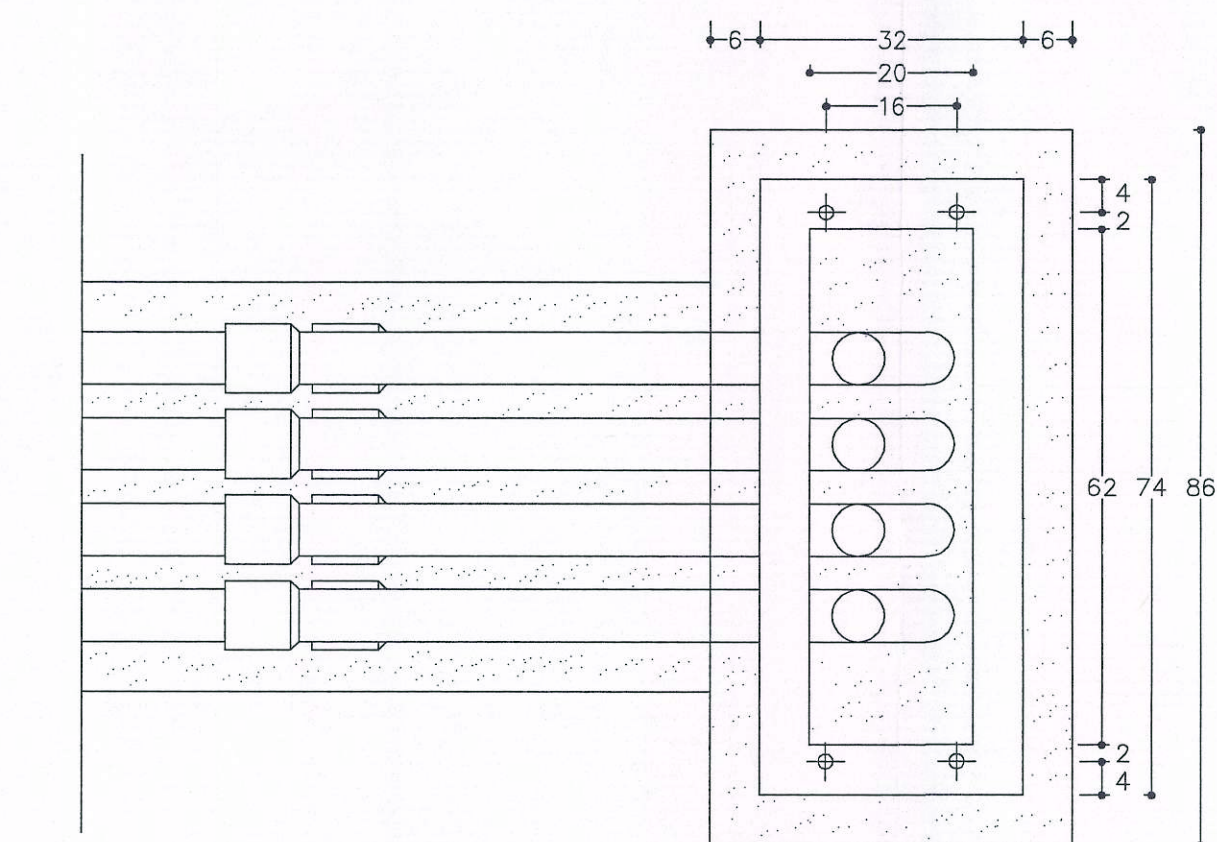
PLANTA
