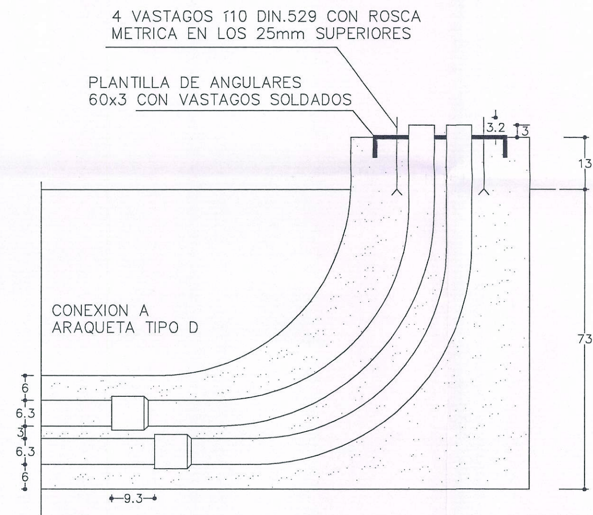
SECCION
