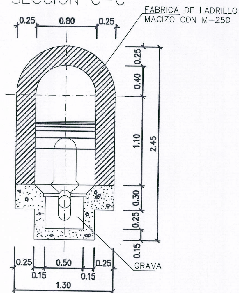
SECCION C-C
