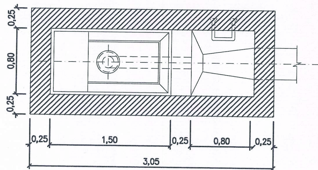
SECCION A-A
