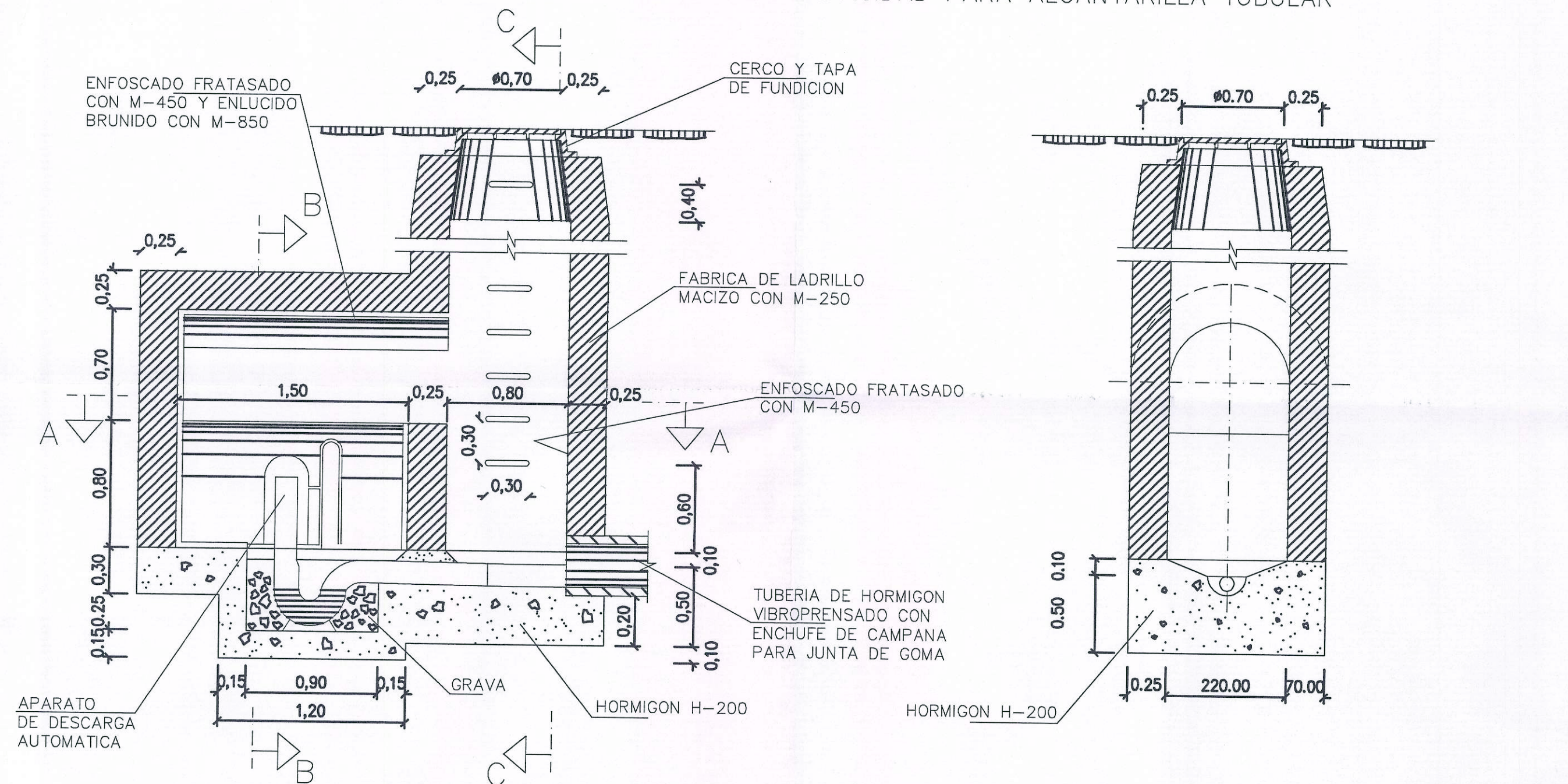
SECCION C-C
