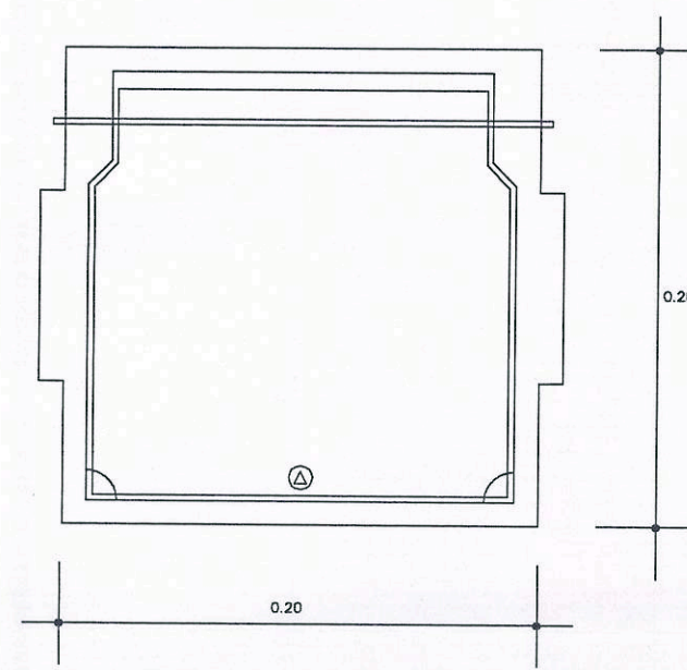
TRAMPILLA LLAVE REGISTRO Escala 1:2
