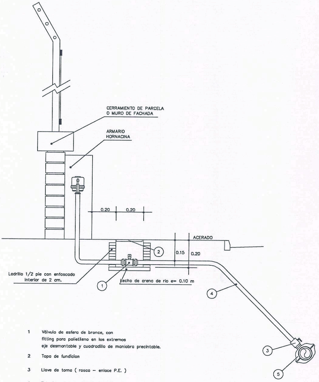
ESQUEMA ACOMETIDA
