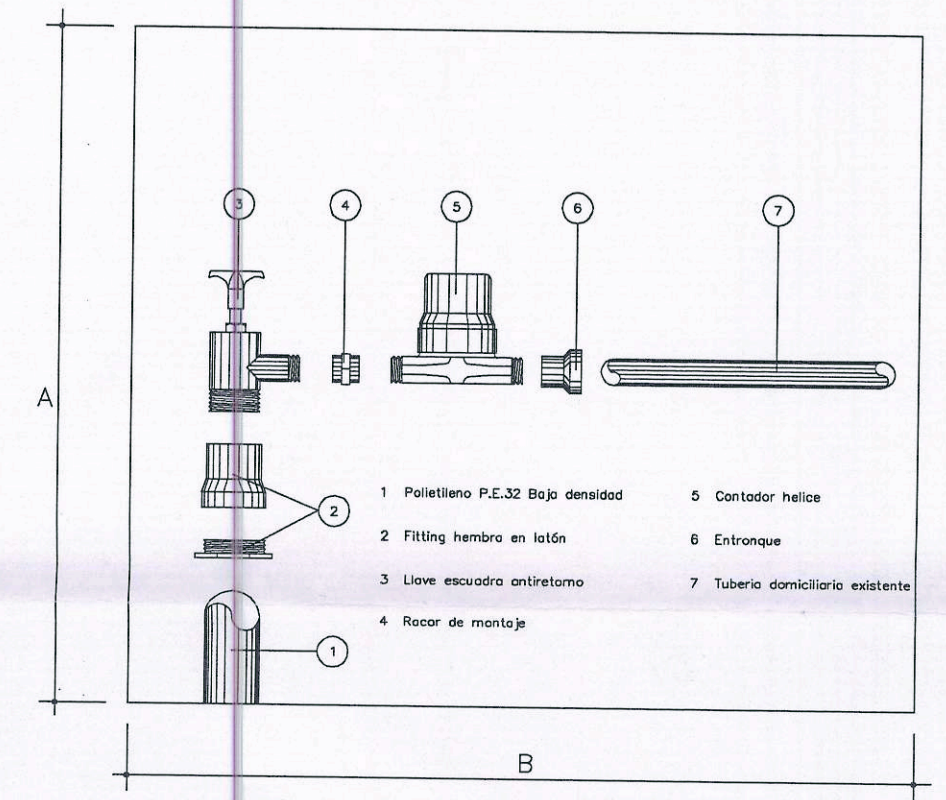
DESPIECE CAJETIN DE CONTADOR Escala 1:2
