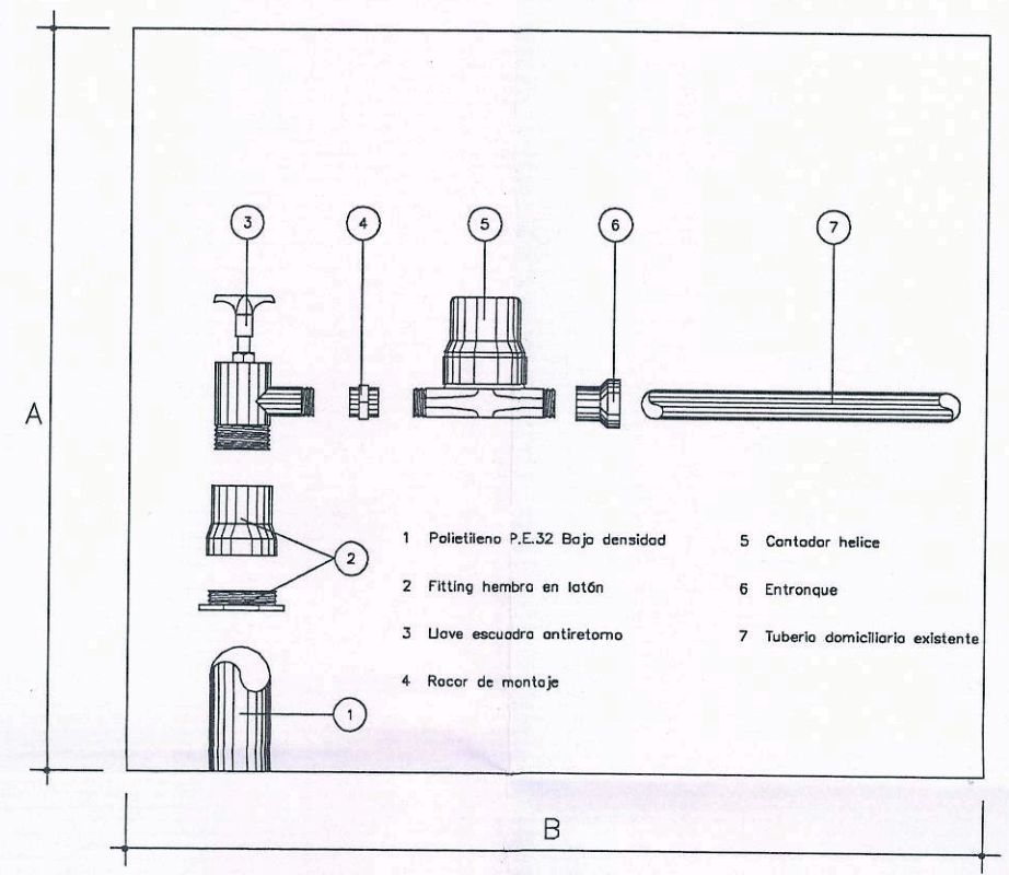
DESPIECE CAJETIN DE CONTADOR Escala 1:2
