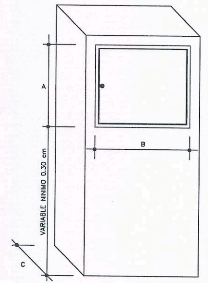
ARMARIO HORNACINA
